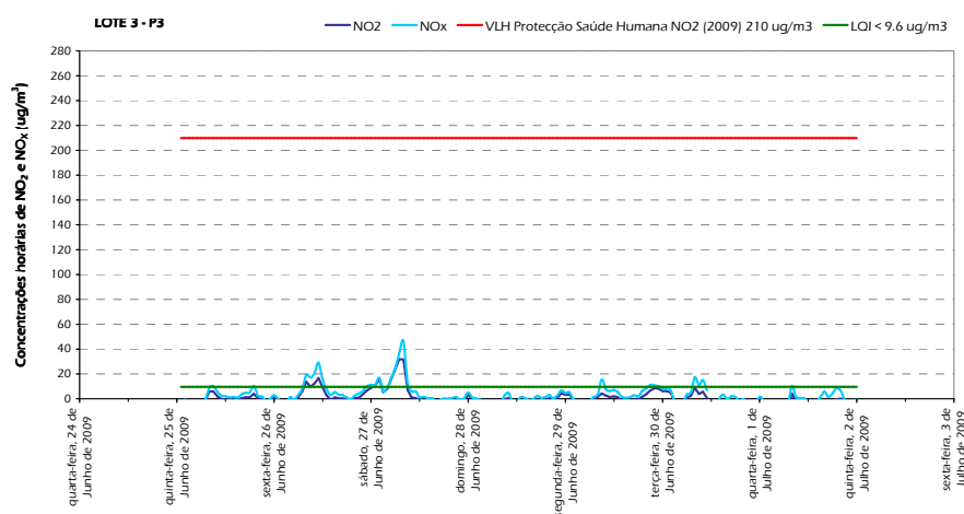
Figura 8 – Gráfico representativo dos resultados horários de Dióxido de Azoto (A) e Óxidos de Azoto (A) obtidos no ponto de medição P3. 1
