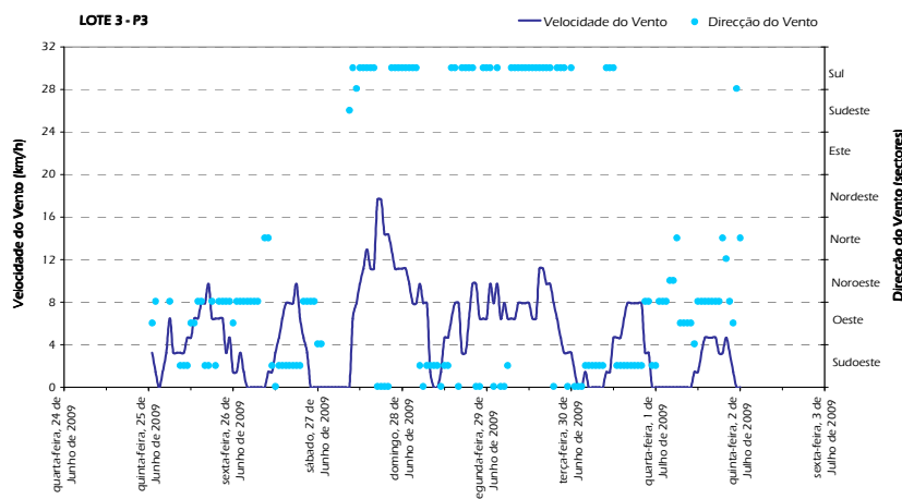
Figura 16 – Variação temporal das médias horárias de direcção e velocidade do vento durante as medições obtidas no ponto de medição P3.
