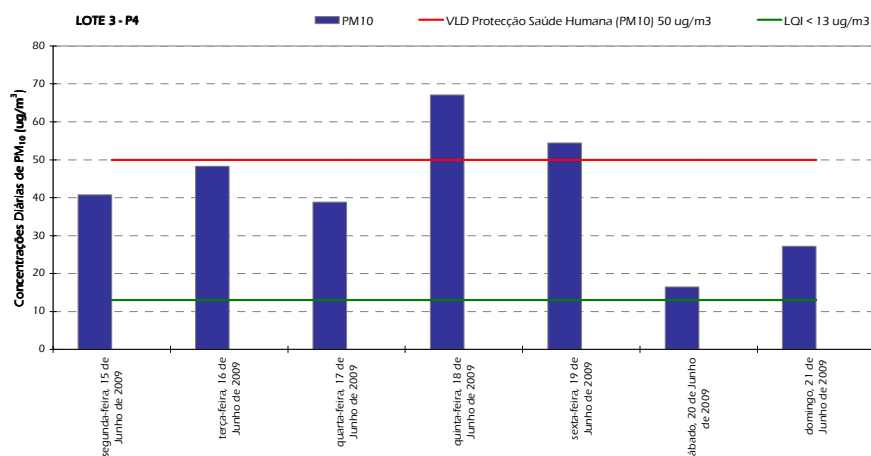
Figura 13 – Gráfico representativo dos resultados diários de PM 10 (A) obtidos no ponto de medição P4 6 .
