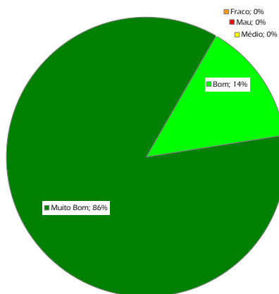
Figura 6 – Gráfico com as percentagens das diferentes classificações observadas durante a campanha de medição realizada em P3.
