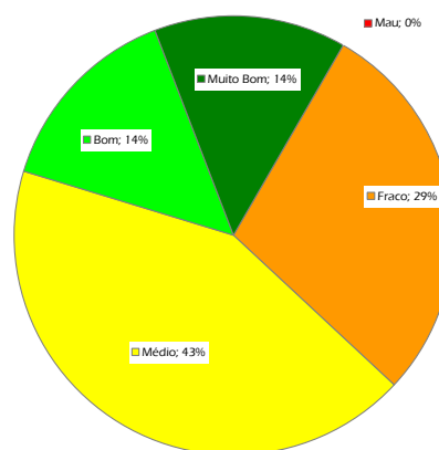
Figura 7 – Gráfico com as percentagens das diferentes classificações observadas durante a campanha de medição realizada em P4.
