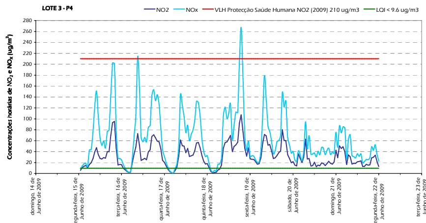
Figura 11 – Gráfico representativo dos resultados horários de Dióxido de Azoto (A) e Óxidos de Azoto (A) obtidos no ponto de medição P4. 4
