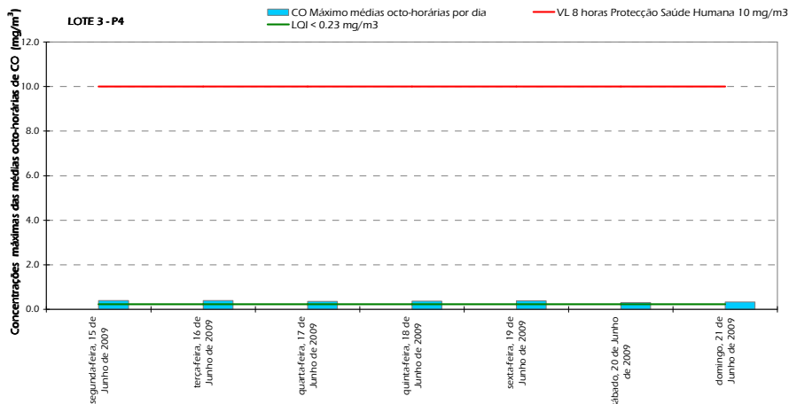
Figura 12 – Gráfico representativo dos resultados máximos octo-horários de Monóxido de Carbono (A) obtidos no ponto de medição P4 5
