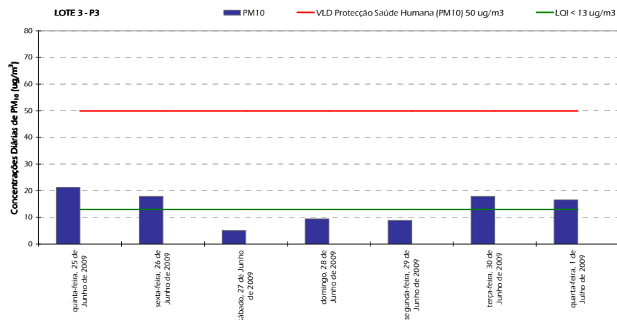
Figura 10 – Gráfico representativo dos resultados diários de PM 10 (A) obtidos no ponto de medição P3 3 .
