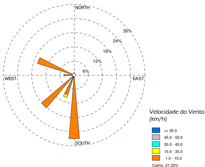
Figura 17 – Rosa de ventos relativa às observações horárias de velocidade e direcção do vento ocorridas no ponto de medição P3.
