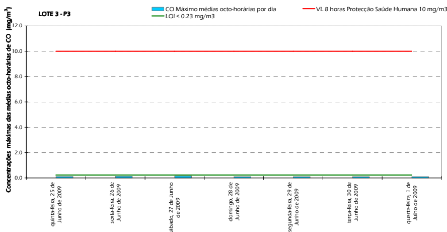
Figura 9 – Gráfico representativo dos resultados máximos octo-horários de Monóxido de Carbono (A) obtidos no ponto de medição P3 2
