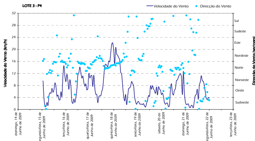
Figura 20 – Variação temporal das médias horárias de direcção e velocidade do vento durante as medições obtidas no ponto de medição P4.
