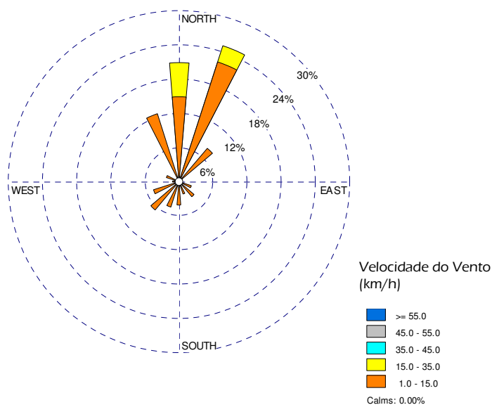
Figura 21 – Rosa de ventos relativa às observações horárias de velocidade e direcção do vento ocorridas no ponto de medição P4.
